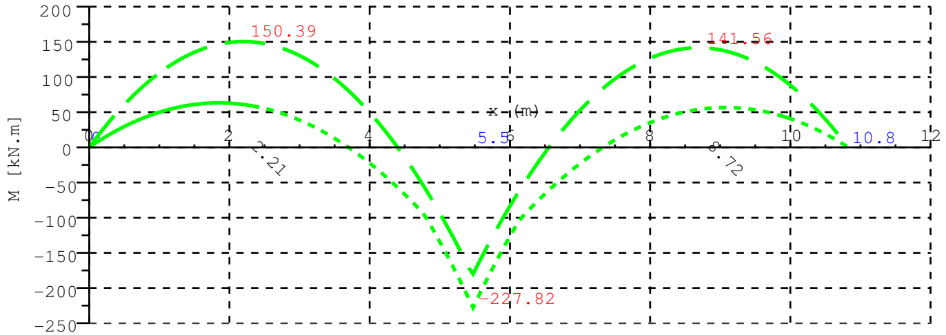
COURBE ENVELOPPE@Moment fl^'chissant [kN.m] (vert)
