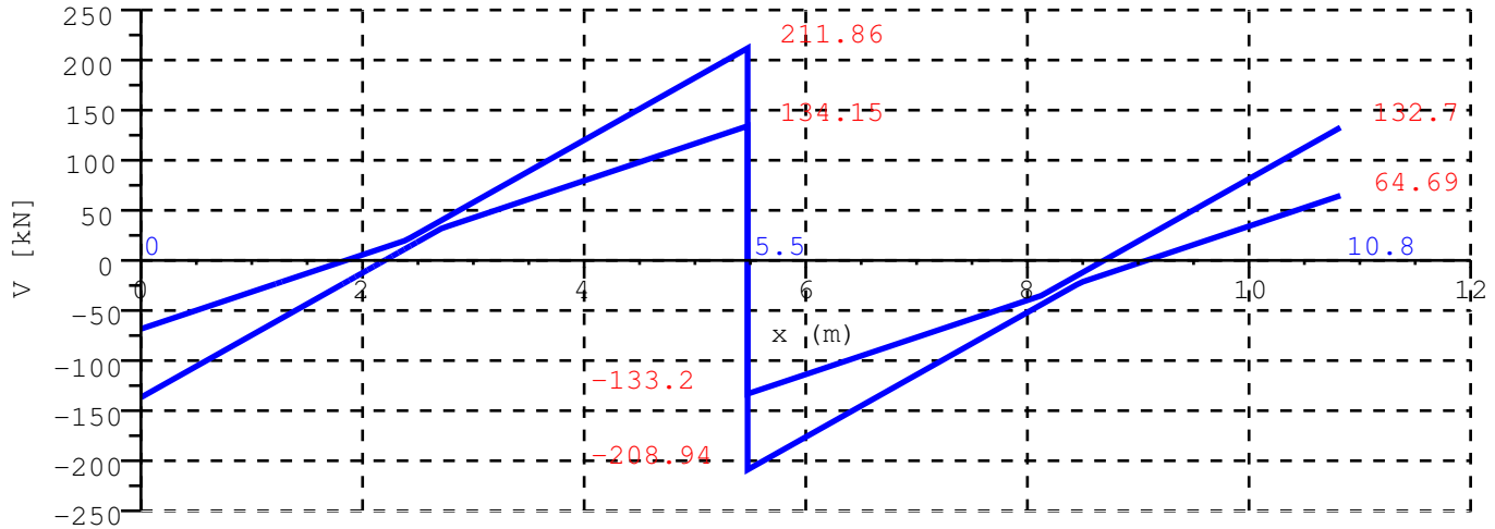
COURBE ENVELOPPE@Effort tranchant [kN] (bleu)
