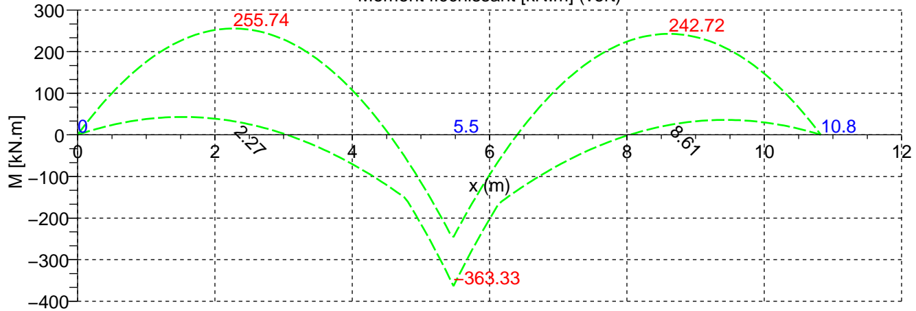
COURBE ENVELOPPE Moment fléchissant [kN.m] (vert)
